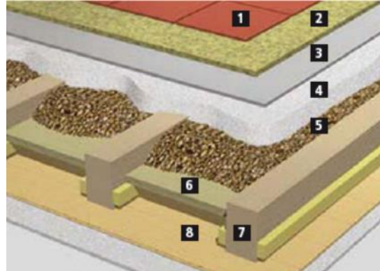
Sanierung Holzbalkendecke mit Fehlboden und vorhandener Auffüllung
