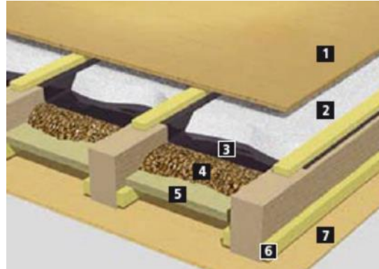
Holzbodenbelag auf Holzbalkendecke mit Fehlboden und vorh. Kies, Lehm oder Schlacke
